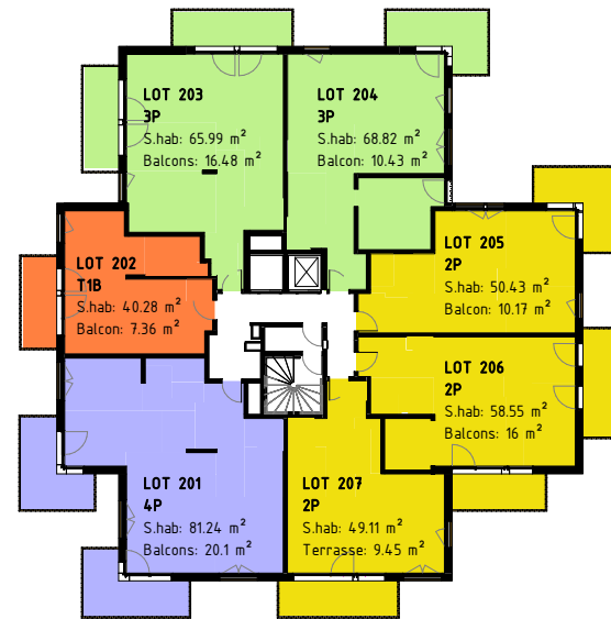
2e étage
