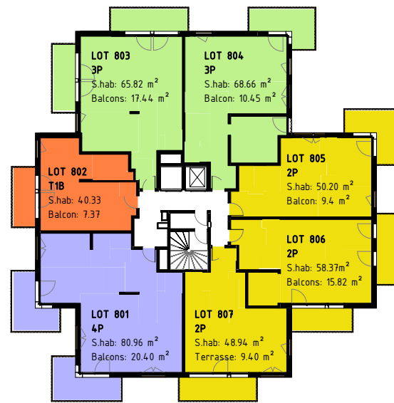
8e étage
