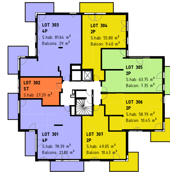
3e étage
