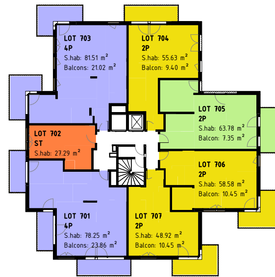
7e étage
