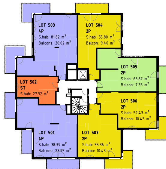
5e étage
