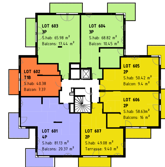
6e étage
